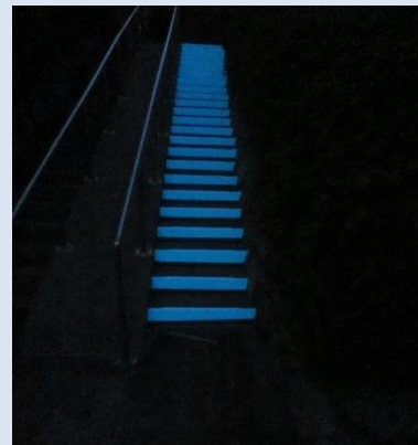
階段の蹴込み部分に蓄光塗料を塗布(夜間) 2014年4月11日午後8時30分撮影
