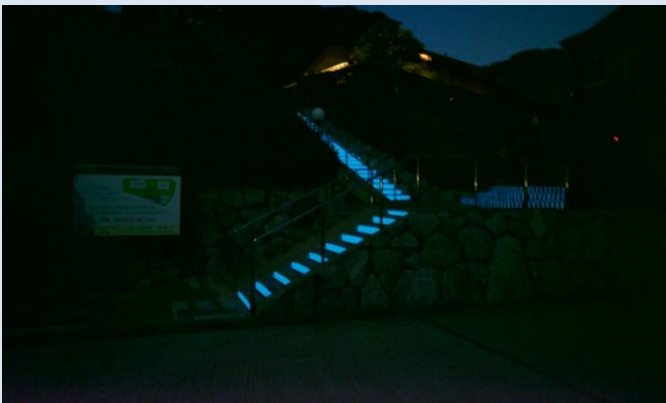
階段の蹴込み部分に蓄光塗料を塗布(夜間) 2014年4月11日午後8時30分撮影
